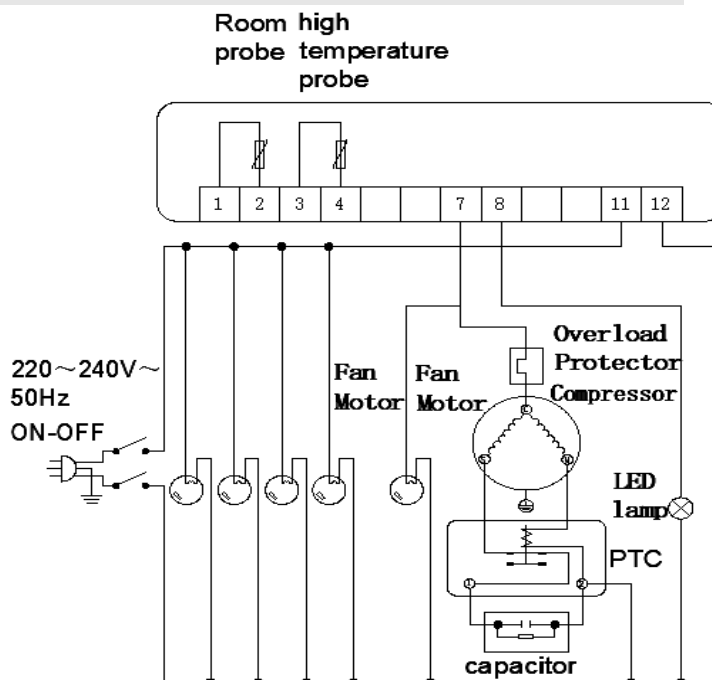
DSFT-470Y/Z/R, DSFT-475Y/Z DSFT-570Y/Z/R, DSFT-575Y/Z
