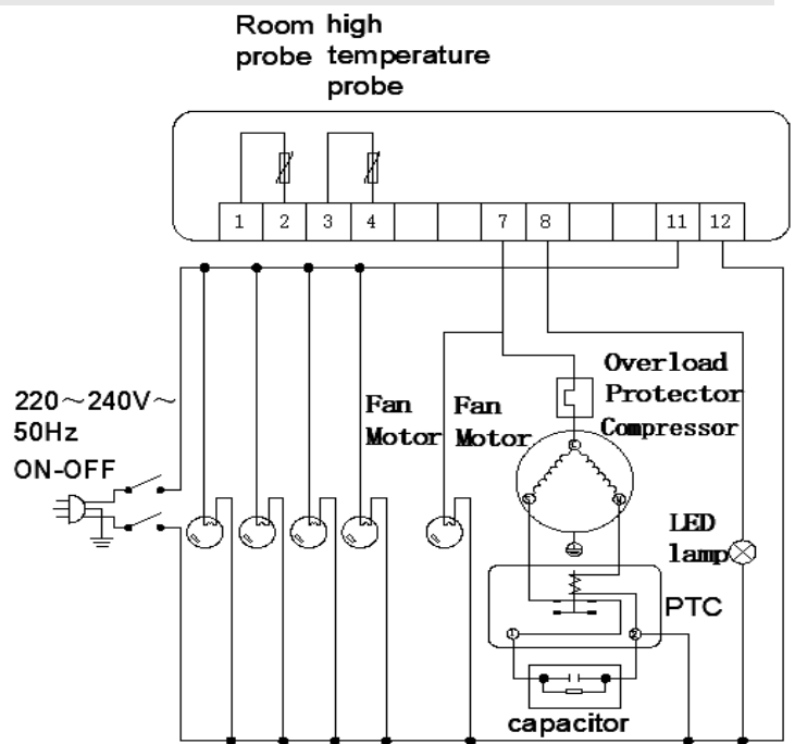
DSFT-470Y/Z/R, DSFT-475Y/Z DSFT-570Y/Z/R, DSFT-575Y/Z
